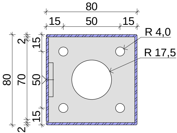
SNITT B-B
